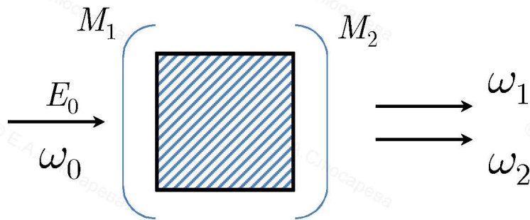
Упрощенная схема параметрического генератора света.
